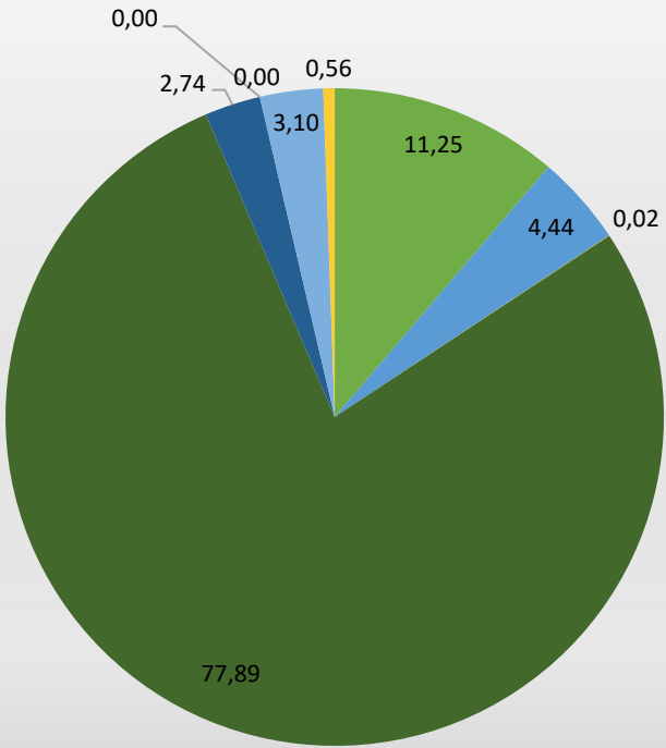
Emissioni di gas serra per fattori di emissione (2024)
